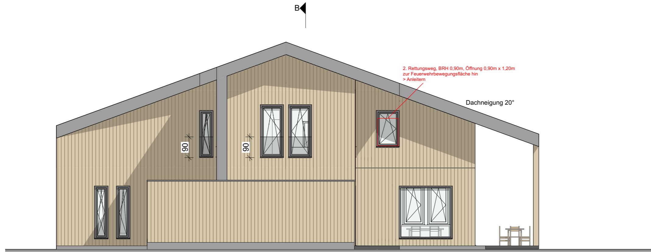
Ansicht WEST
